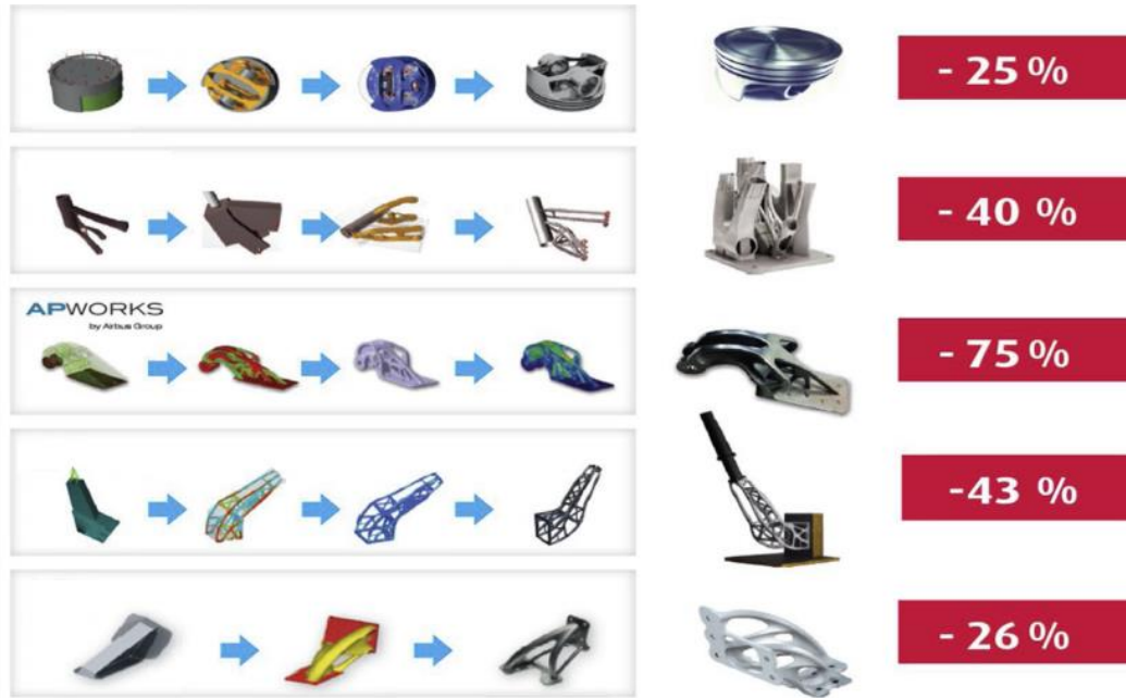
Şekil 2. Topoloji optimizasyonu uygulanan parçalar ve ağırlık kayıp oranları [15]
