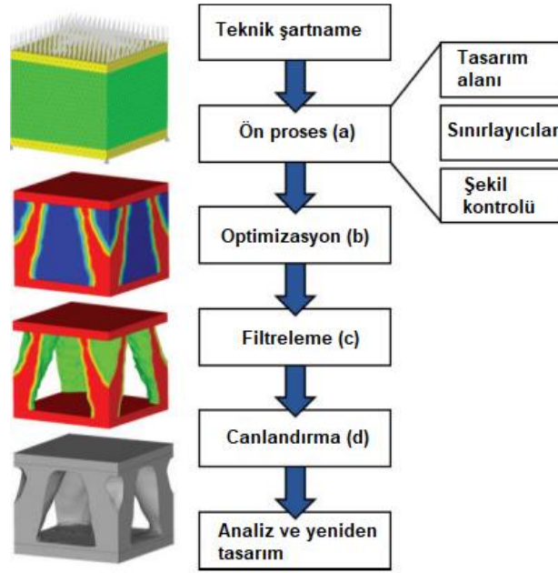
Şekil 1. Topoloji optimizasyonu işlem basamakları [9]
