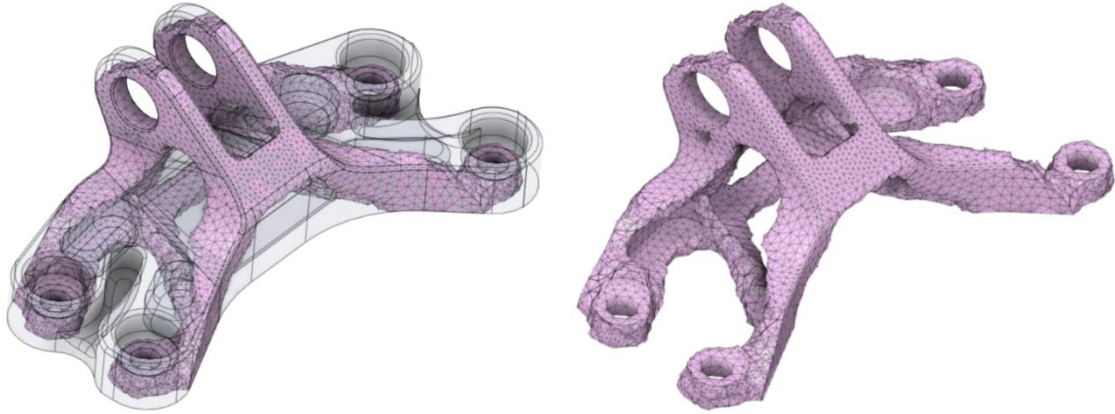
Şekil 5. Ağırlığı optimize edilen en uygun braket görüntüsü
